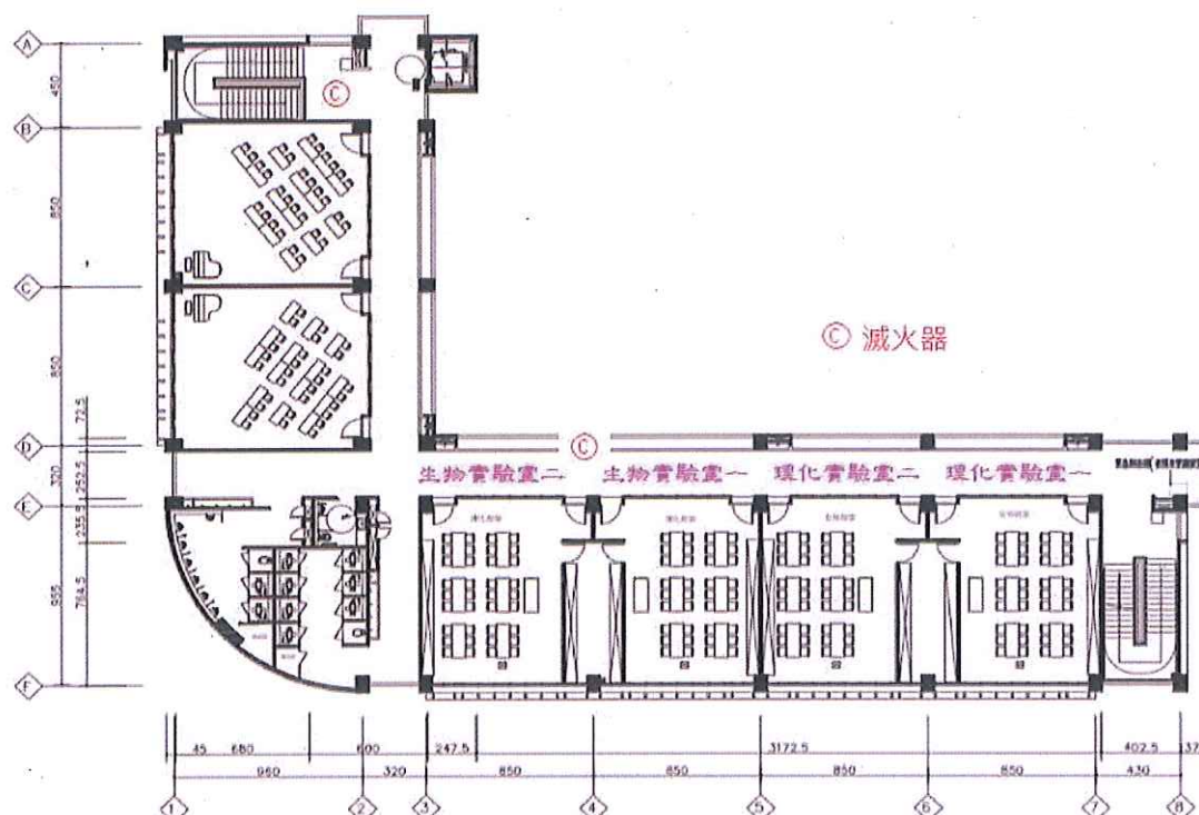
平面圖
