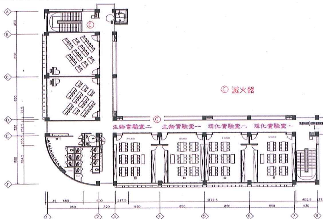
平面圖
